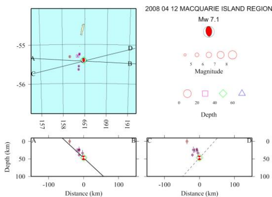
図 1 2008 年 4 月 12 日にマッコリー島地域で発生した地震 (Mw7.1) の余震分布と震源断層面 (左下図の実線)。
