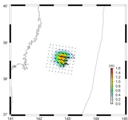
図 2 2011 年 3 月 9 日に三陸沖で発生した地震
