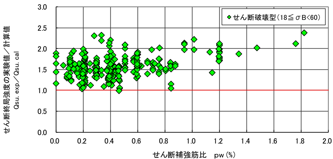
図 4.6.30 せん断強度 (実験値/計算値：基準下限式) - せん断補強筋比関係 (せん断破壊型)
