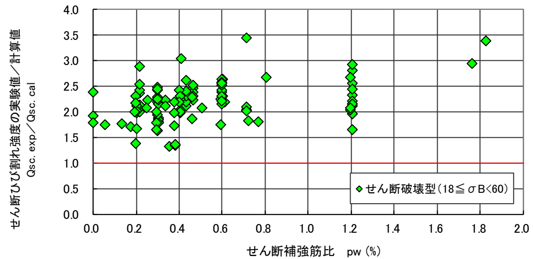
図 4.6.24 せん断ひび割れ強度 (実験値/計算値) - せん断補強筋比関係 (せん断破壊型)
