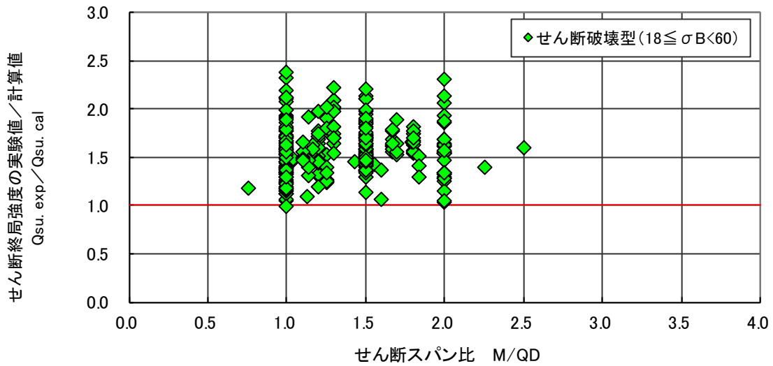
図 4.6.27 せん断強度（実験値／計算値：基準下限式）－せん断スパン比関係（せん断破壊型）
