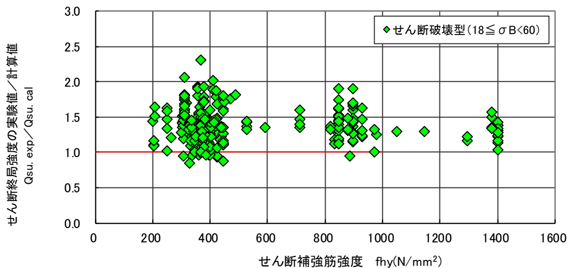
図 4.6.38 せん断強度（実験値／計算値：基準平均値式）－せん断補強筋強度関係（せん断破壊型）
