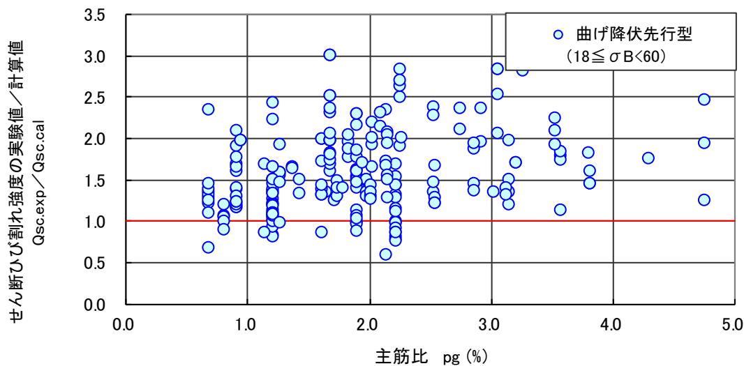
図 4.5.23 せん断ひび割れ強度（実験値／計算値）－主筋比関係（曲げ降伏先行型）
