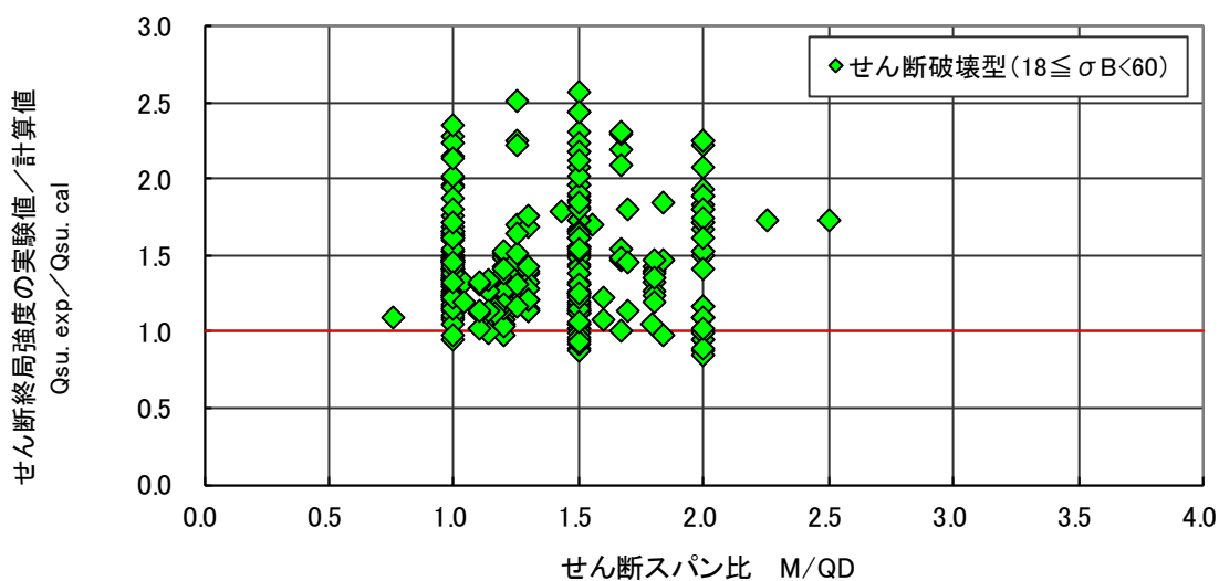
図 4.6.41 せん断強度（実験値／計算値：靱性指針式）－せん断スパン比関係（せん断破壊型）
