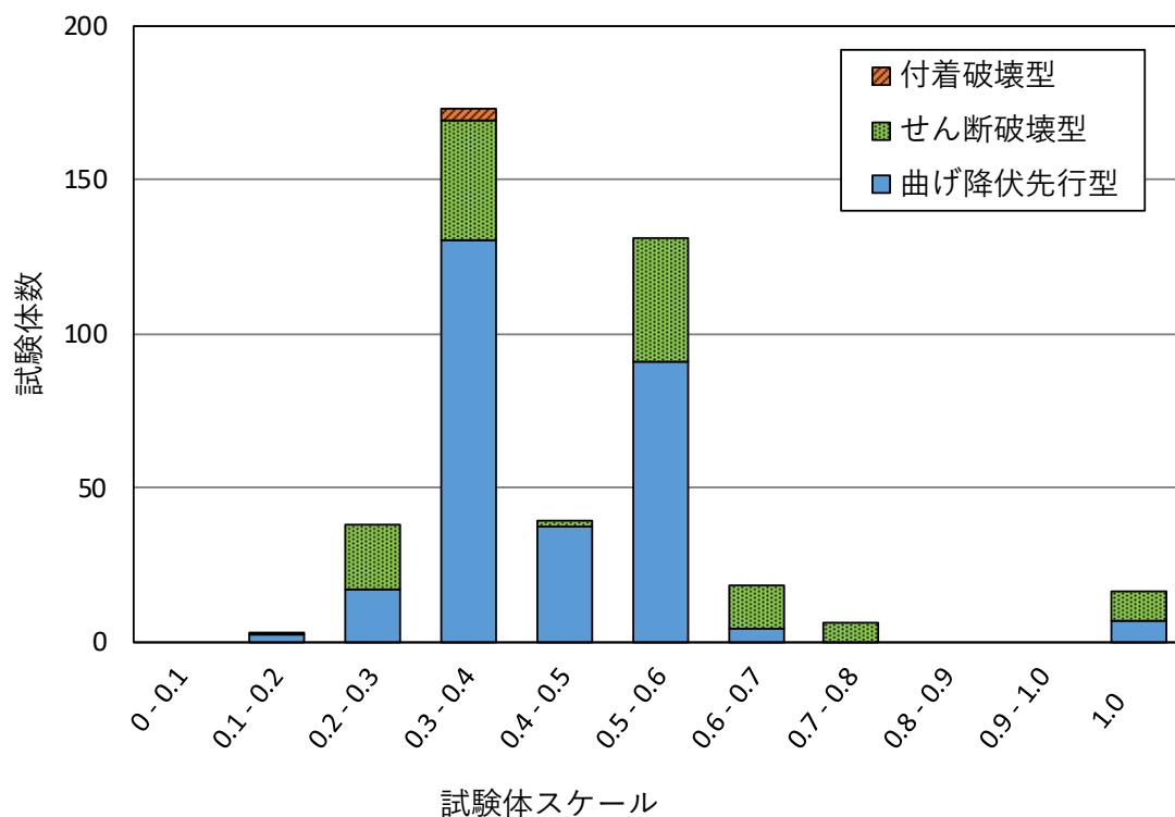
図 4.2.12 収集データの頻度分布 (試験体スケール) (横軸は区間下限値以上から区間上限値未満)
