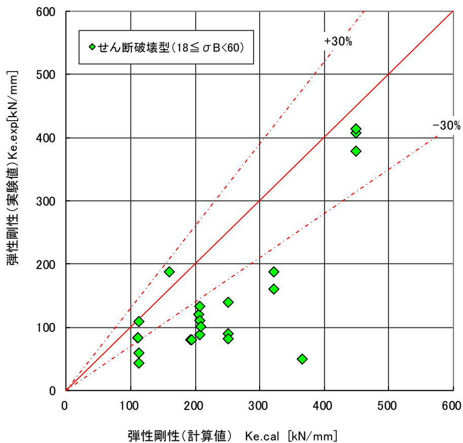
図 4.6.7 弾性剛性の実験値と計算値の関係
