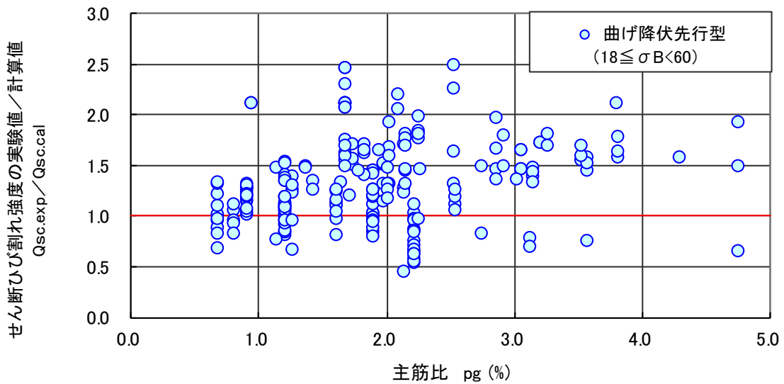
図 4.5.17 セン断ひび割れ強度（実験値／計算値）－主筋比関係（曲げ降伏先行型）
