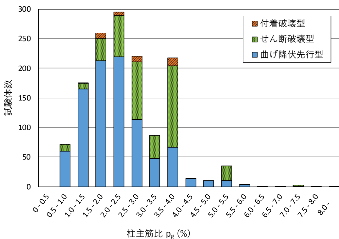
図 4.2.5 収集データの頻度分布 (柱主筋比) (横軸は区間下限値以上から区間上限値未満)
