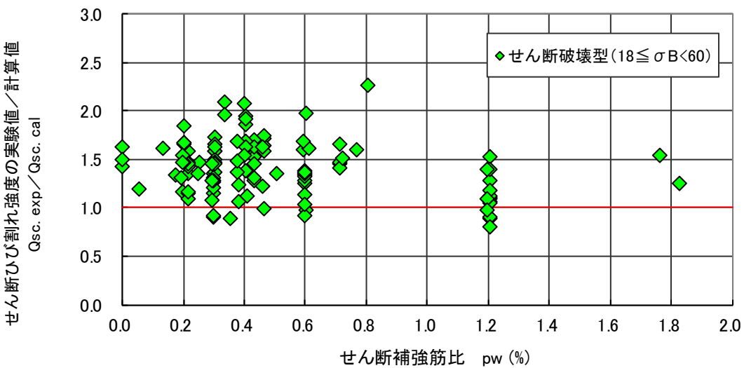
図 4.6.18 せん断ひび割れ強度（実験値／計算値）－せん断補強筋比関係（せん断破壊型）
