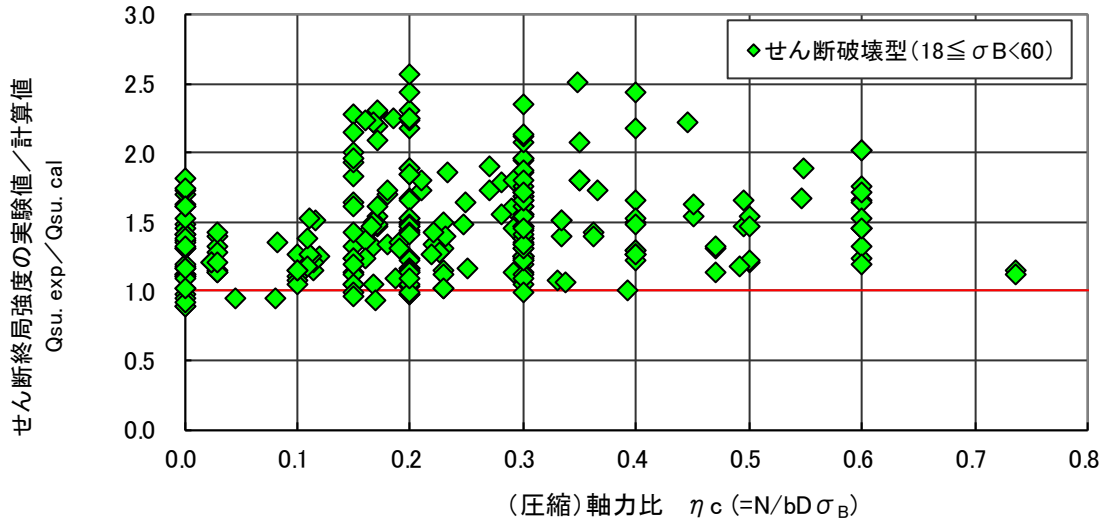
図 4.6.43 せん断強度（実験値／計算値：靱性指針式）－圧縮軸力比関係（せん断破壊型）
