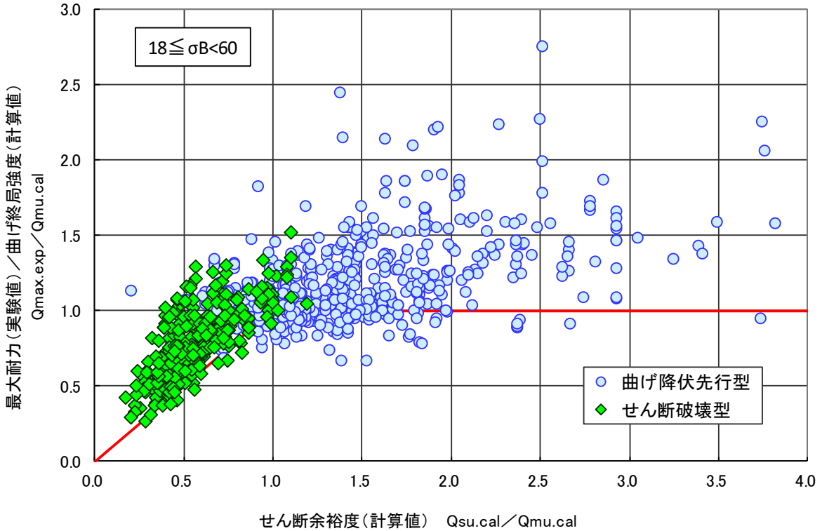
図 4.6.47 最大耐力(実験値) / 曲げ終局強度(計算値) - せん断余裕度(計算値) 関係 (曲げ降伏先行型+せん断破壊型データ) せん断強度式は靱性指針 (4.5.8)式
