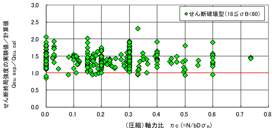
図 4.6.36 せん断強度（実験値／計算値：基準平均値式）－圧縮軸力比関係（せん断破壊型）
