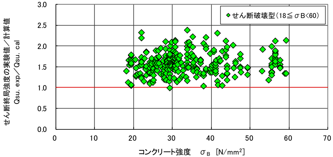
図 4.6.26 せん断強度（実験値／計算値：基準下限式）－コンクリート強度関係（せん断破壊型）
