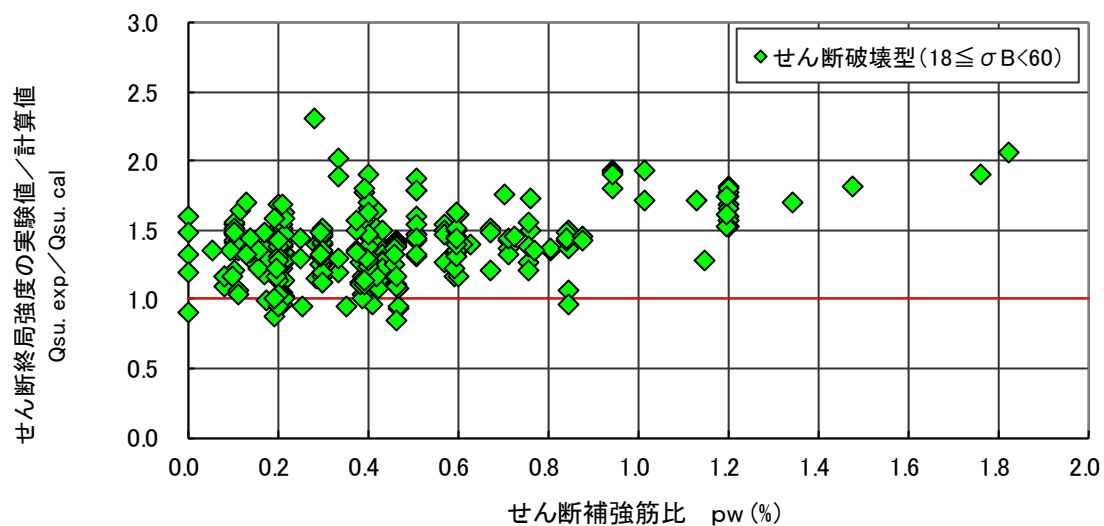
図 4.6.37 せん断強度（実験値／計算値：基準平均値式）－せん断補強筋比関係（せん断破壊型）
