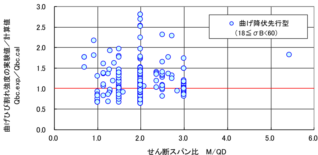
図 4.5.3 曲げひび割れ強度（実験値／計算値）－せん断スパン比関係（曲げ降伏先行型）
