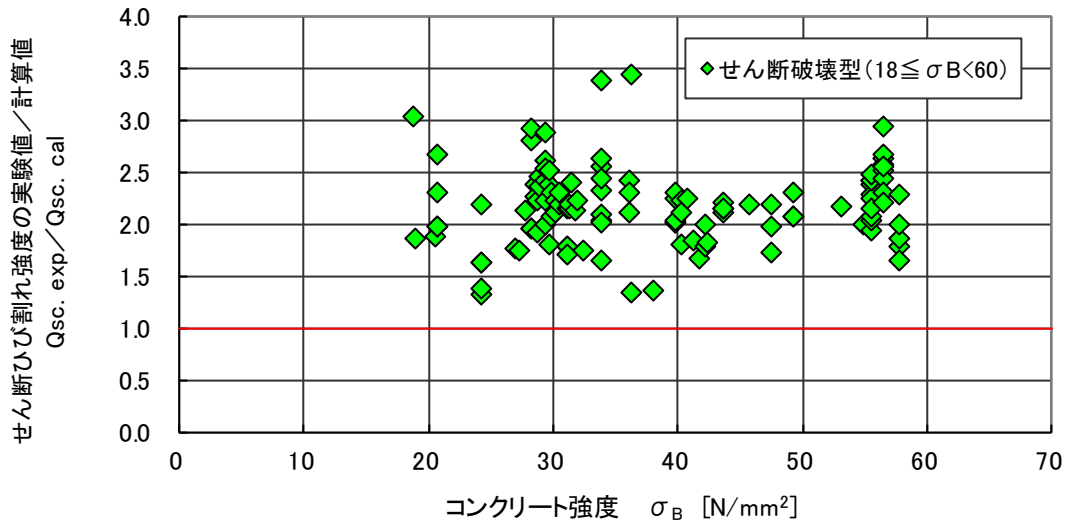
図 4.6.20 せん断ひび割れ強度（実験値／計算値）－コンクリート強度関係（せん断破壊型）
