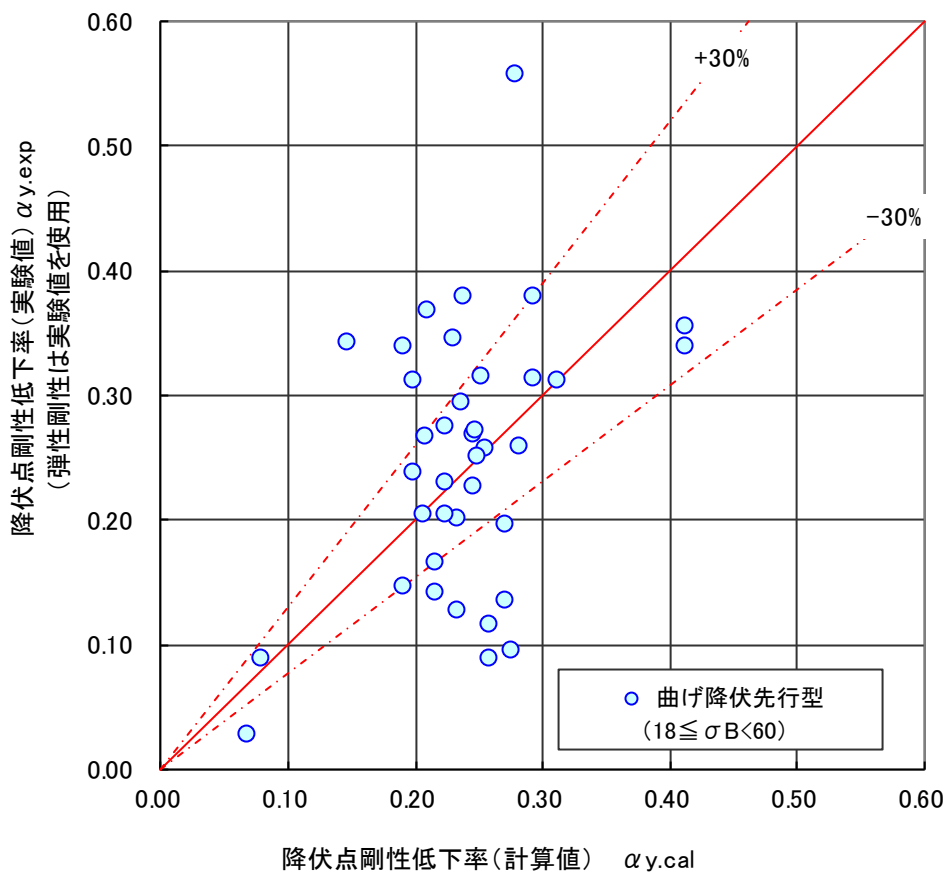
図 4.5.40 降伏点剛性低下率の実験値と計算値の比較
