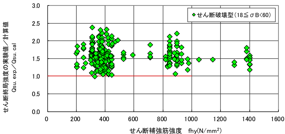
図 4.6.31 せん断強度 (実験値/計算値：基準下限式) - せん断補強筋強度関係 (せん断破壊型)
