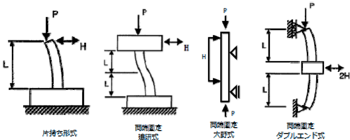
図 4.1.4 加力形式
