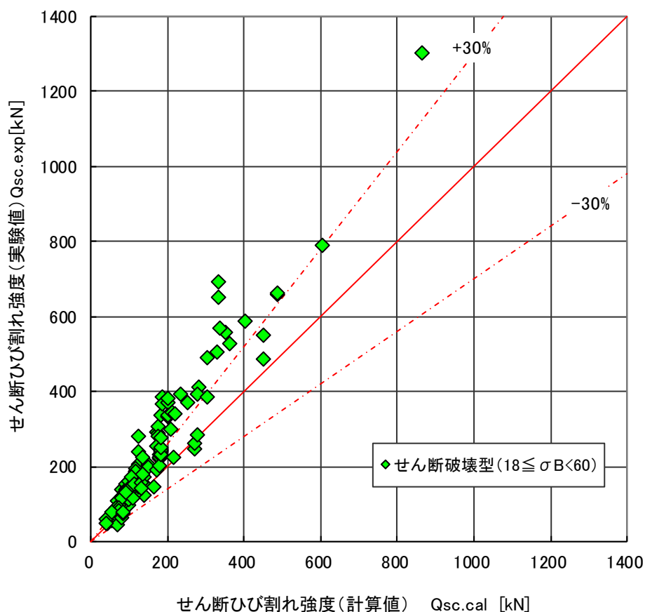
図 4.6.13 せん断ひび割れ強度の実験値と計算値の比較（せん断破壊型）
