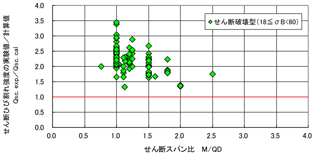
図 4.6.21 せん断ひび割れ強度（実験値／計算値）－せん断スパン比関係（せん断破壊型）
