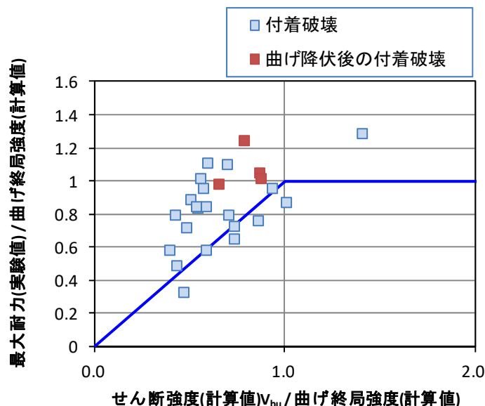
図 4.7.11 せん断強度 V_{bu} と最大耐力（実験値）の関係（ \tau_{bu}/\tau_y < 1 の試験体）
