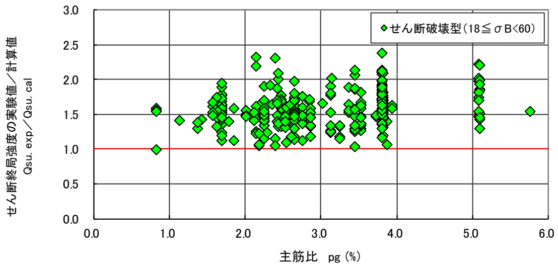
図 4.6.28 せん断強度（実験値／計算値：基準下限式）－主筋比関係（せん断破壊型）
