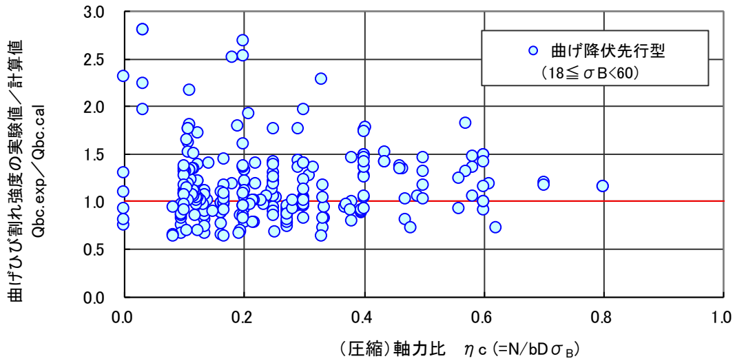
図 4.5.6 曲げひび割れ強度（実験値／計算値）－圧縮軸力比関係（曲げ降伏先行型）
