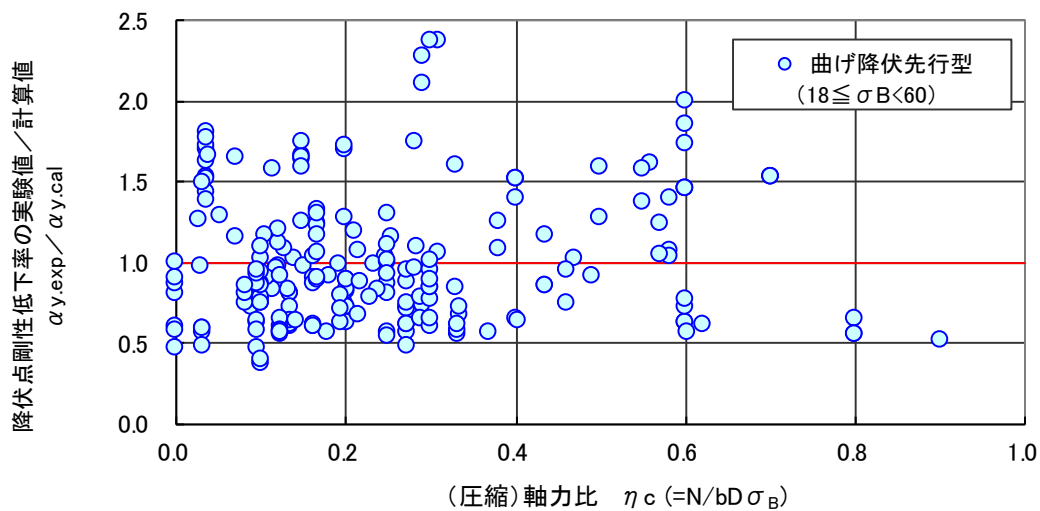
図 4.5.45 降伏点剛性低下率（実験値／計算値）－圧縮軸力比関係（曲げ降伏先行型）
