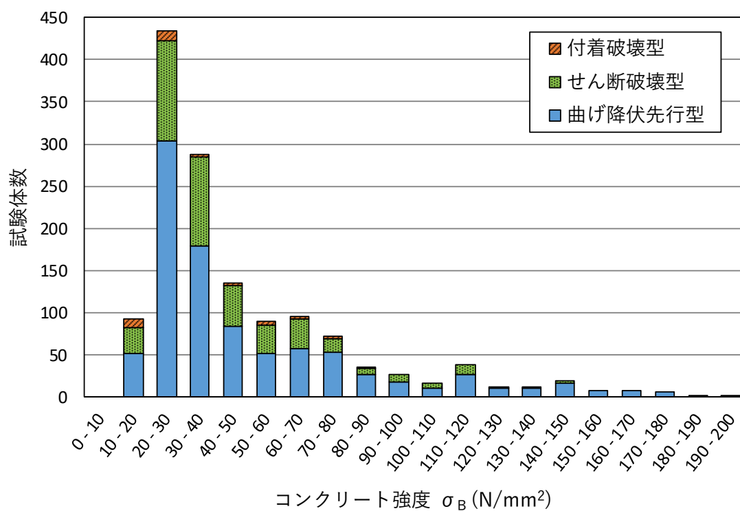
図 4.2.3 収集データの頻度分布 (コンクリート強度)
