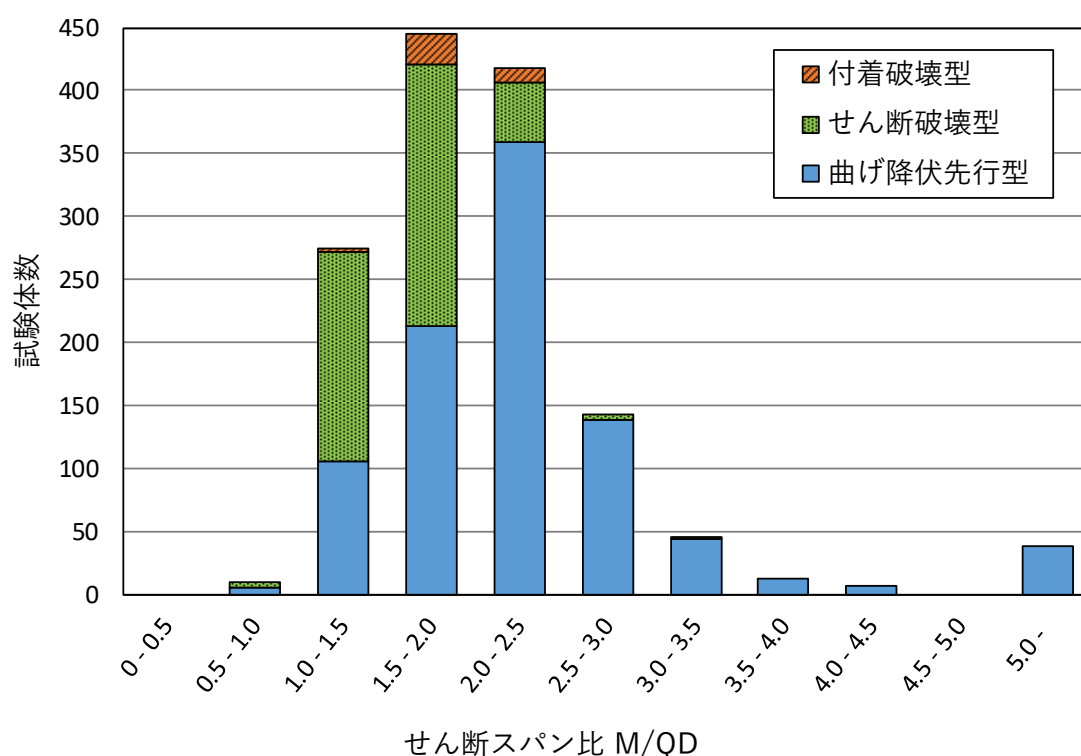
図 4.2.13 収集データの頻度分布 (せん断スパン比)
