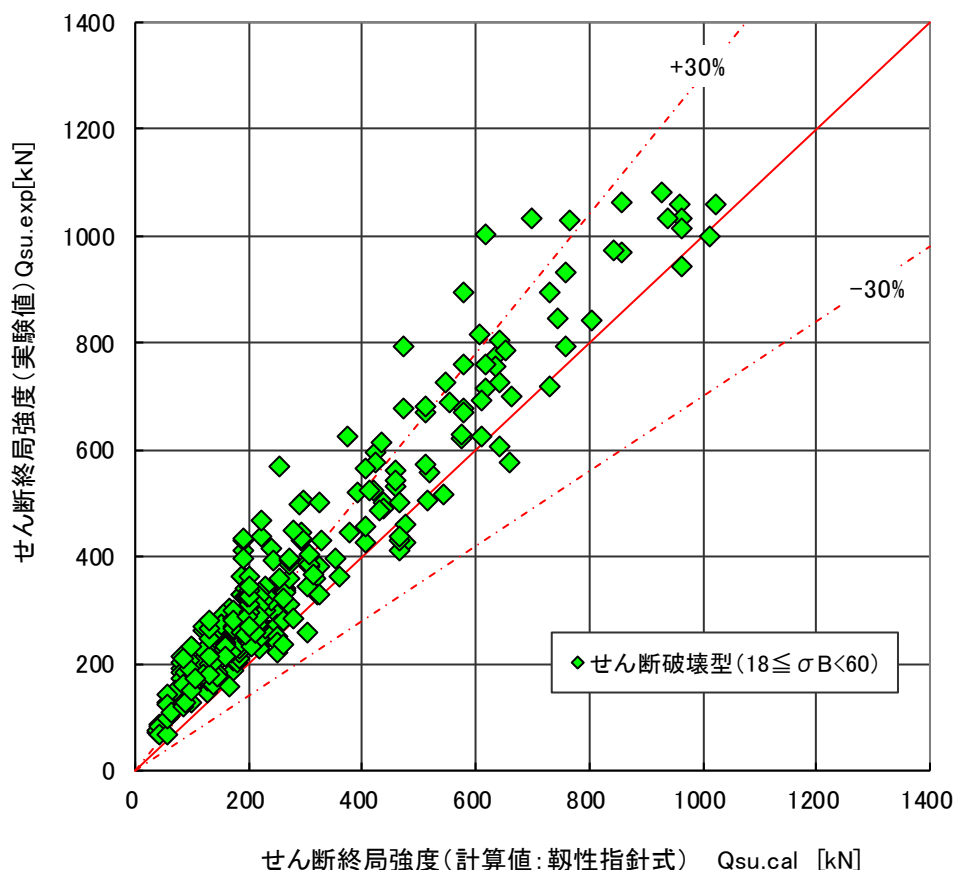
図 4.6.39 せん断強度の実験値と計算値②（靱性指針式）の比較（せん断破壊型）
