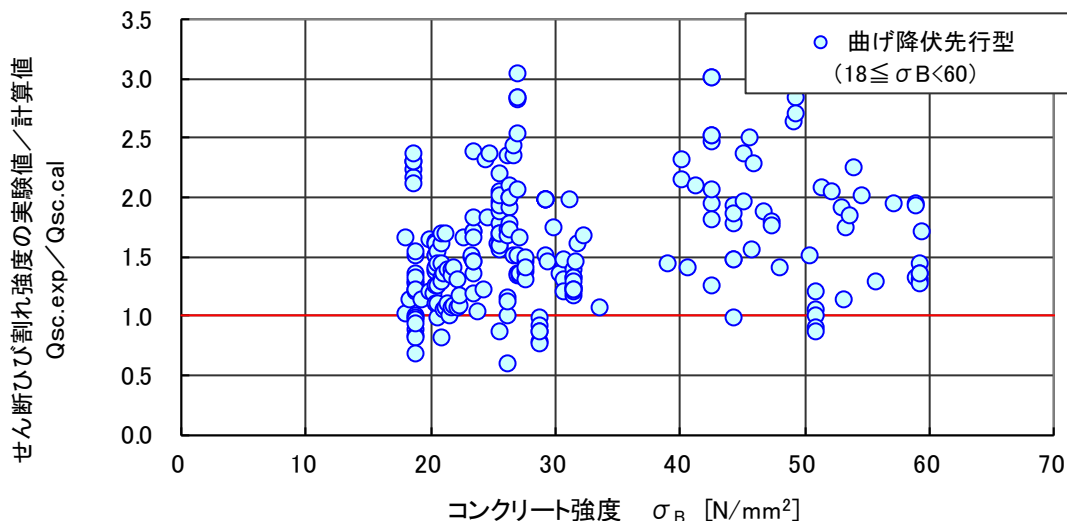
図 4.5.21 せん断ひび割れ強度（実験値／計算値）－コンクリート強度関係（曲げ降伏先行型）
