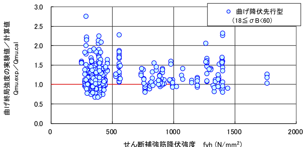
図 4.5.33 曲げ終局強度（実験値／計算値）－せん断補強筋降伏強度関係（曲げ降伏先行型）
