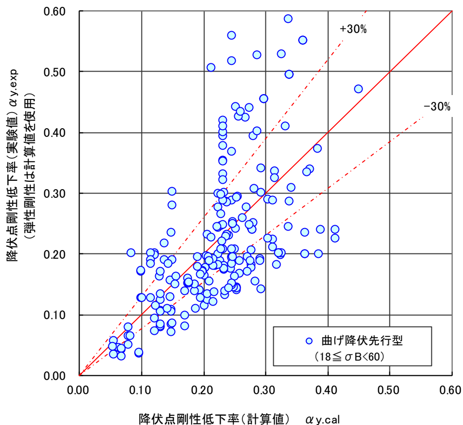
図 4.5.39 降伏点剛性低下率の実験値と計算値の比較
