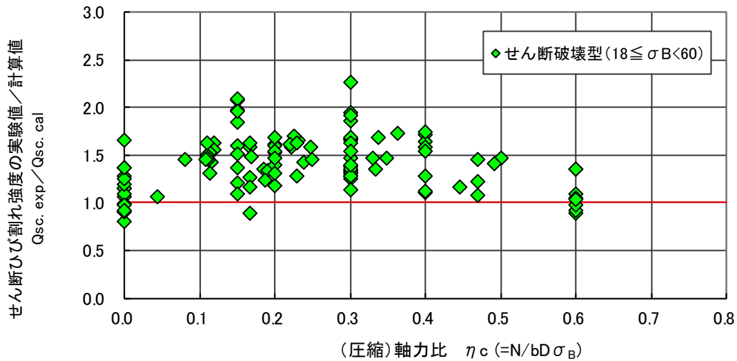
図 4.6.17 せん断ひび割れ強度（実験値／計算値）－圧縮軸力比関係（せん断破壊型）
