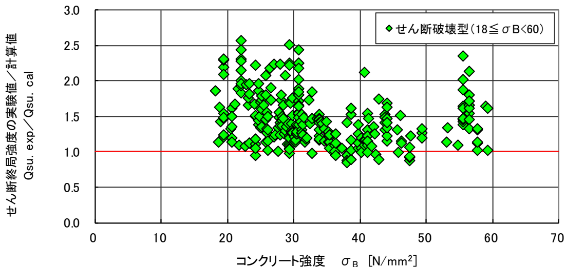
図 4.6.40 せん断強度（実験値／計算値：靱性指針式）－コンクリート強度関係（せん断破壊型）
