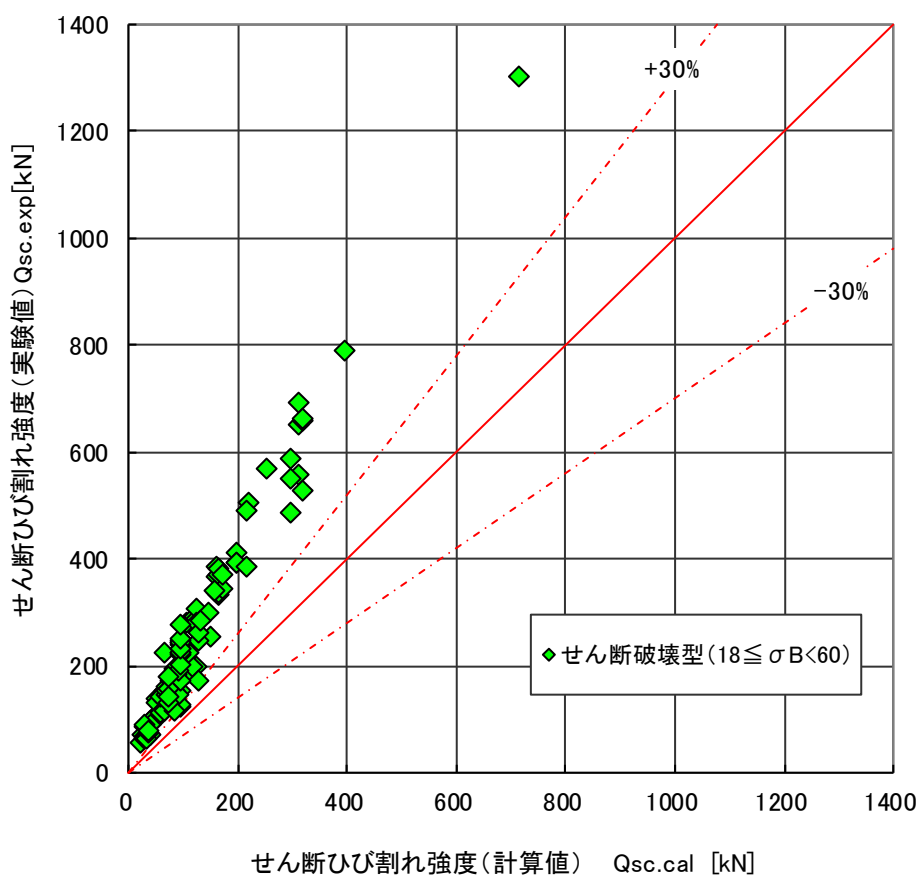
図 4.6.19 せん断ひび割れ強度の実験値と計算値 (靱性指針式) の比較 (せん断破壊型)
