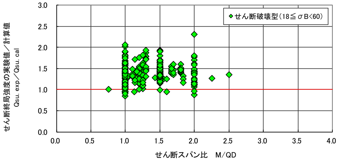
図 4.6.34 せん断強度（実験値／計算値：基準平均値式）－せん断スパン比関係（せん断破壊型）
