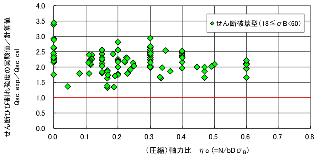
図 4.6.23 せん断ひび割れ強度 (実験値/計算値) - 圧縮軸力比関係 (せん断破壊型)
