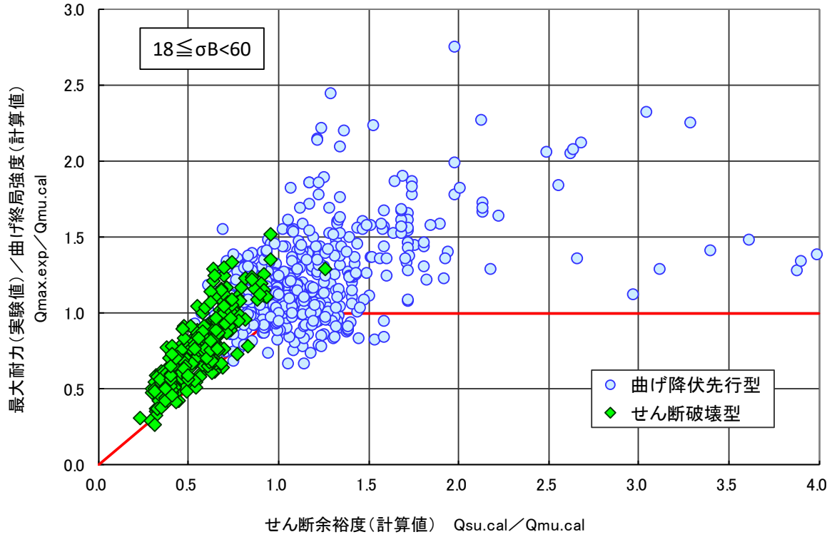
図 4.6.46 最大耐力(実験値) / 曲げ終局強度(計算値) - せん断余裕度(計算値) 関係 (曲げ降伏先行型+せん断破壊型データ) せん断強度式は基準平均値式 (4.5.7)式
