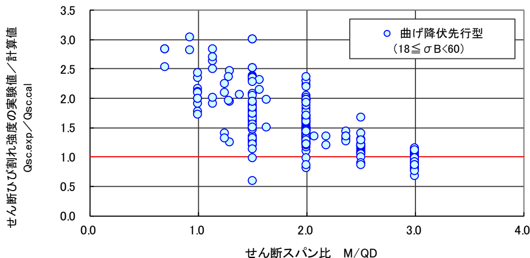
図 4.5.22 せん断ひび割れ強度（実験値／計算値）－せん断スパン比関係（曲げ降伏先行型）
