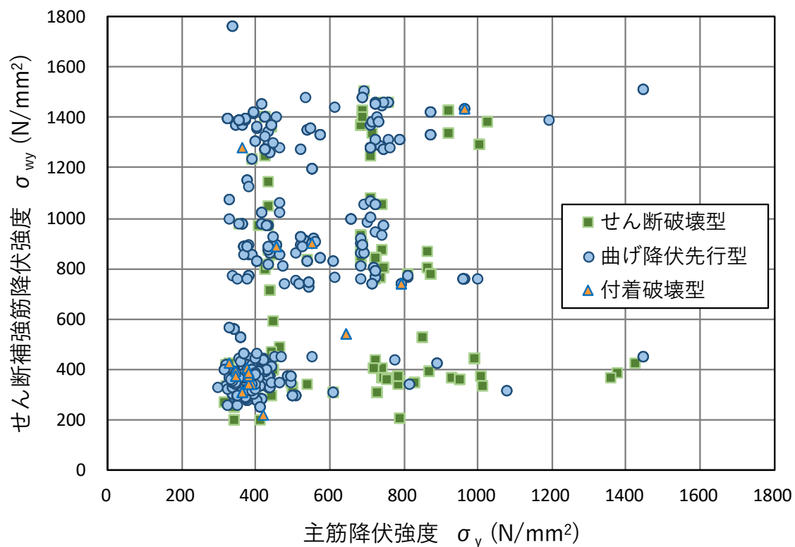
図 4.2.11 収集データの頻度分布 (主筋降伏強度-せん断補強筋降伏強度の関係)
