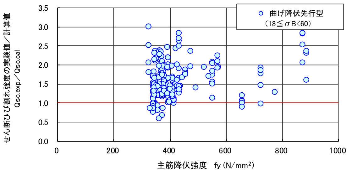
図 4.5.24 せん断ひび割れ強度（実験値／計算値）－主筋降伏強度関係（曲げ降伏先行型）
