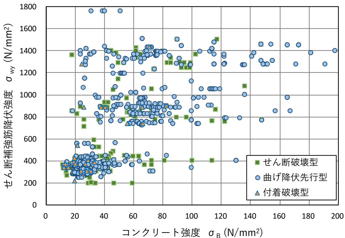
図 4.2.10 収集データの頻度分布 (コンクリート強度-せん断補強筋降伏強度の関係)
