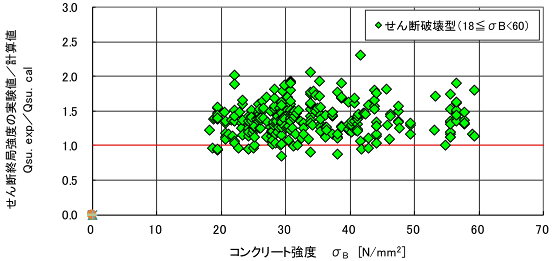
図 4.6.33 せん断強度（実験値／計算値：基準平均値式）－コンクリート強度関係（せん断破壊型）
