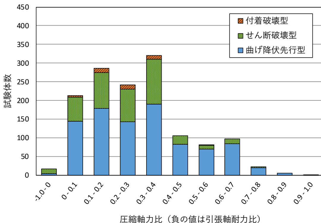
図 4.2.14 引用した試験体で使った軸力比
