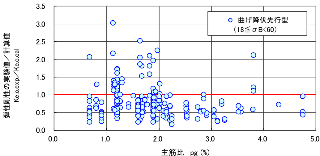
図 4.5.11 弾性剛性（実験値／計算値）－主筋比関係（曲げ降伏先行型）
