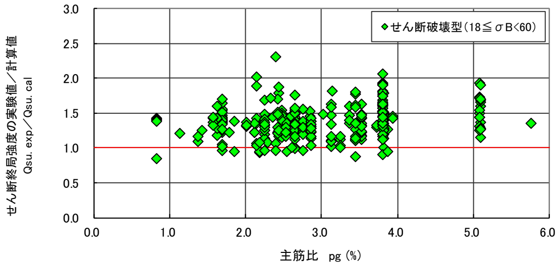
図 4.6.35 （実験値／計算値：基準平均値式）－主筋比関係（せん断破壊型）
