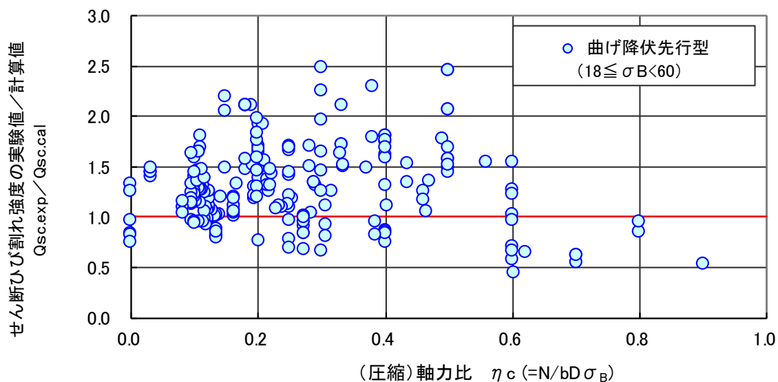
図 4.5.19 せん断ひび割れ強度（実験値／計算値）－圧縮軸力比関係（曲げ降伏先行型）
