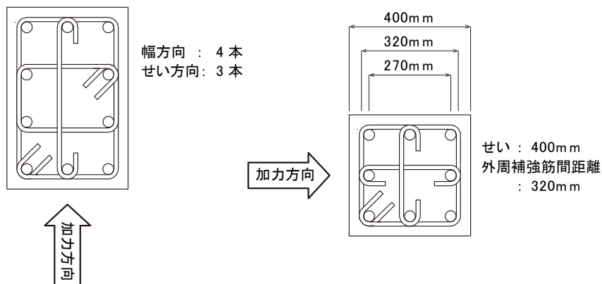
図 4.1.1 補強筋有効本数
