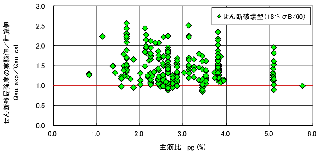
図 4.6.42 せん断強度（実験値／計算値：靱性指針式）－主筋比関係（せん断破壊型）
