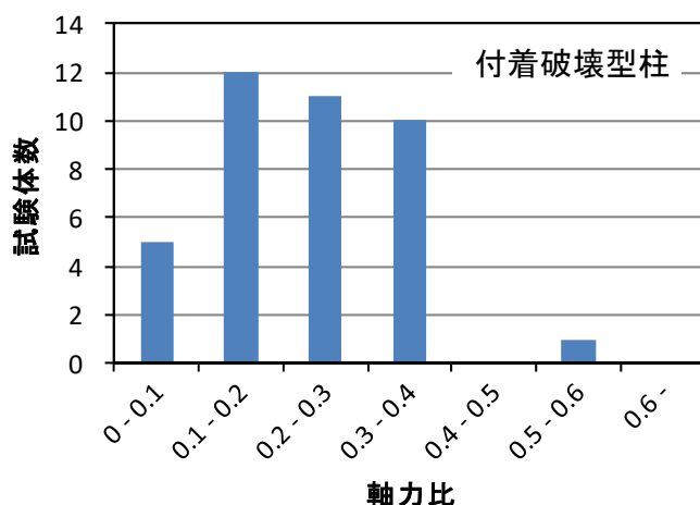
図 4.7.7 軸力比
