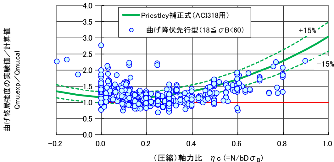
図 4.5.31 曲げ終局強度（実験値／計算値）－圧縮軸力比関係（曲げ降伏先行型）
