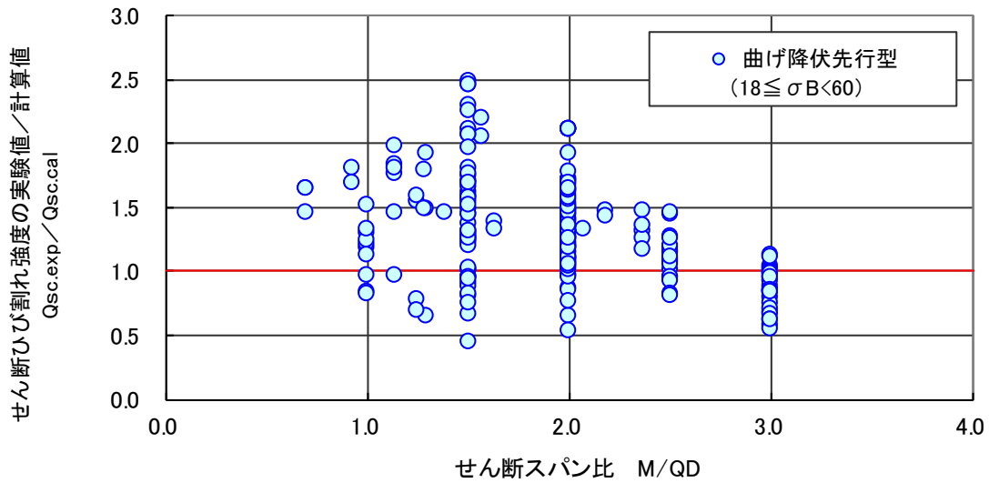
図 4.5.16 セン断ひび割れ強度（実験値／計算値）－せん断スパン比関係（曲げ降伏先行型）
