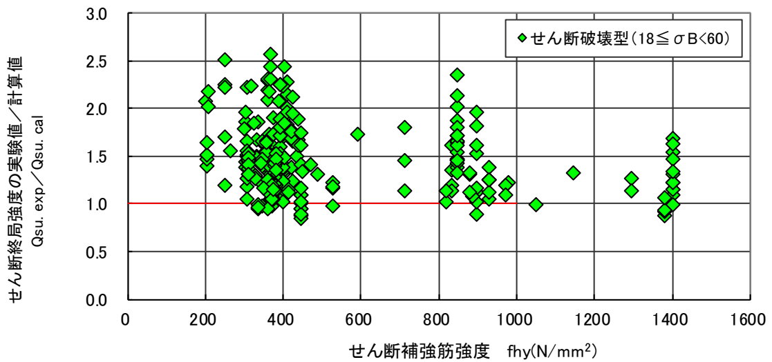
図 4.6.45 せん断強度（実験値／計算値：靱性指針式）－せん断補強筋強度関係（せん断破壊型）
