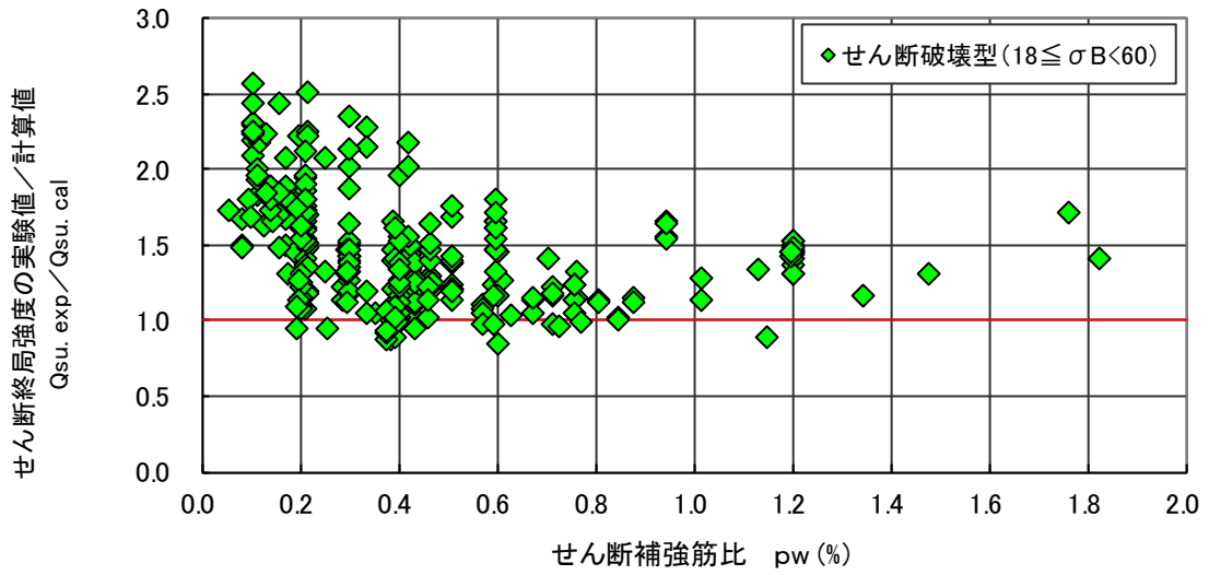
図 4.6.44 せん断強度（実験値／計算値：靱性指針式）－せん断補強筋比関係（せん断破壊型）
