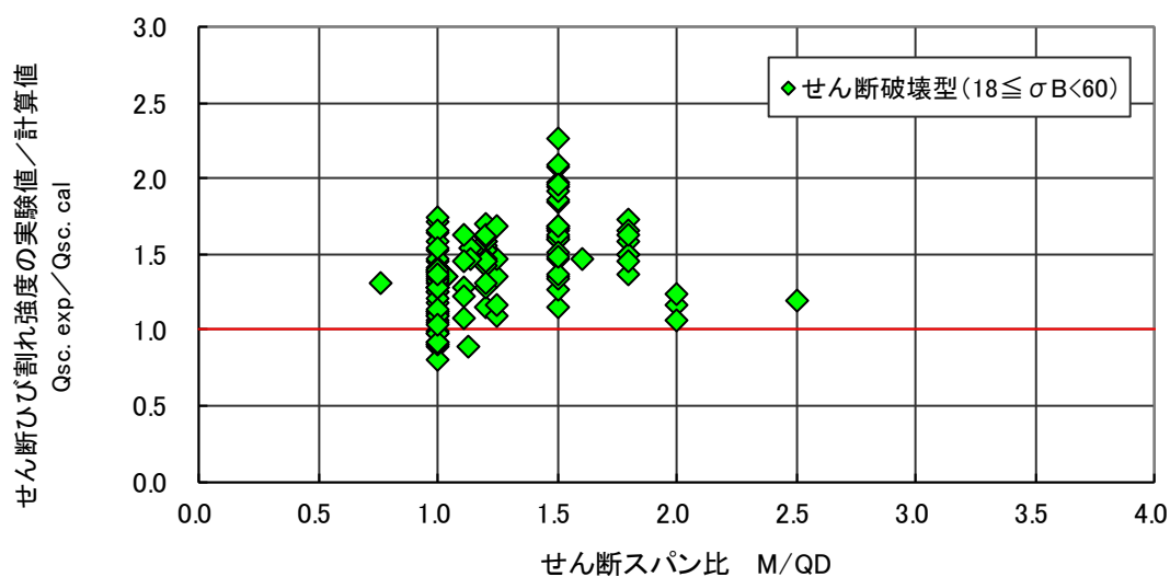
図 4.6.15 せん断ひび割れ強度（実験値／計算値）－せん断スパン比関係（せん断破壊型）
