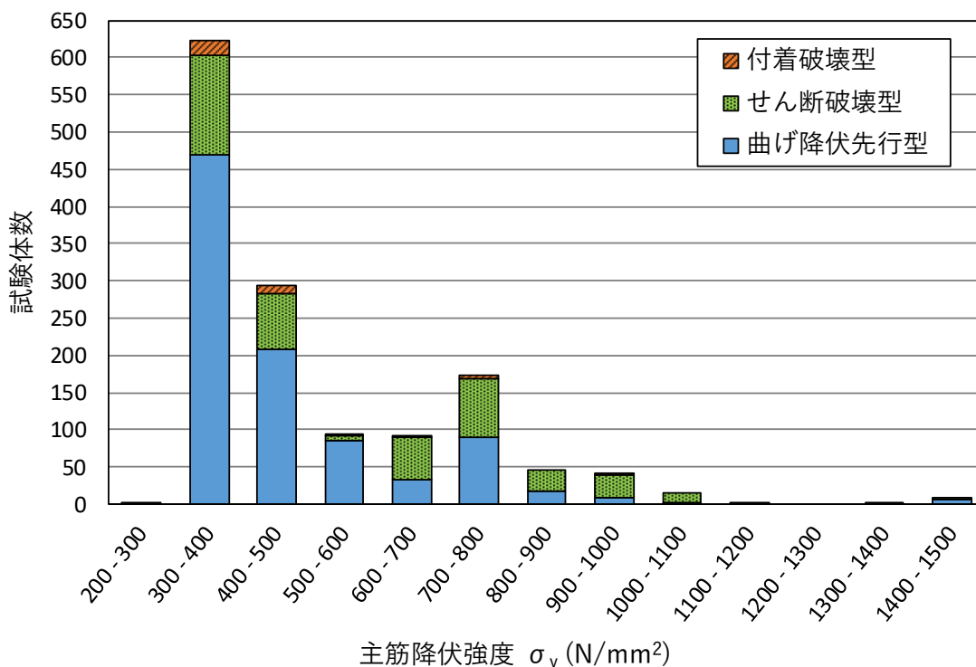
図 4.2.4 収集データの頻度分布 (主筋降伏強度) (横軸は区間下限値以上から区間上限値未満)
