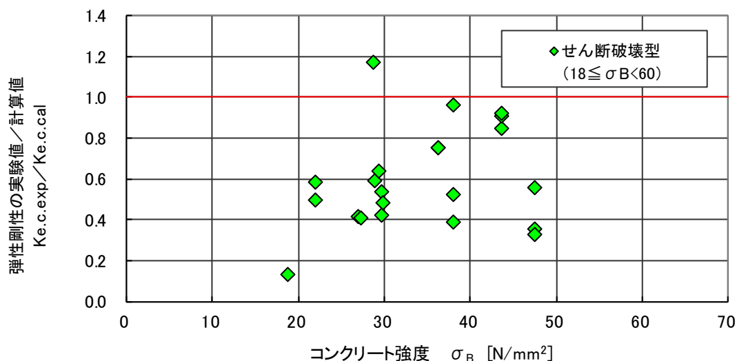
図 4.6.8 弾性剛性（実験値／計算値）－コンクリート強度関係（せん断破壊型）
