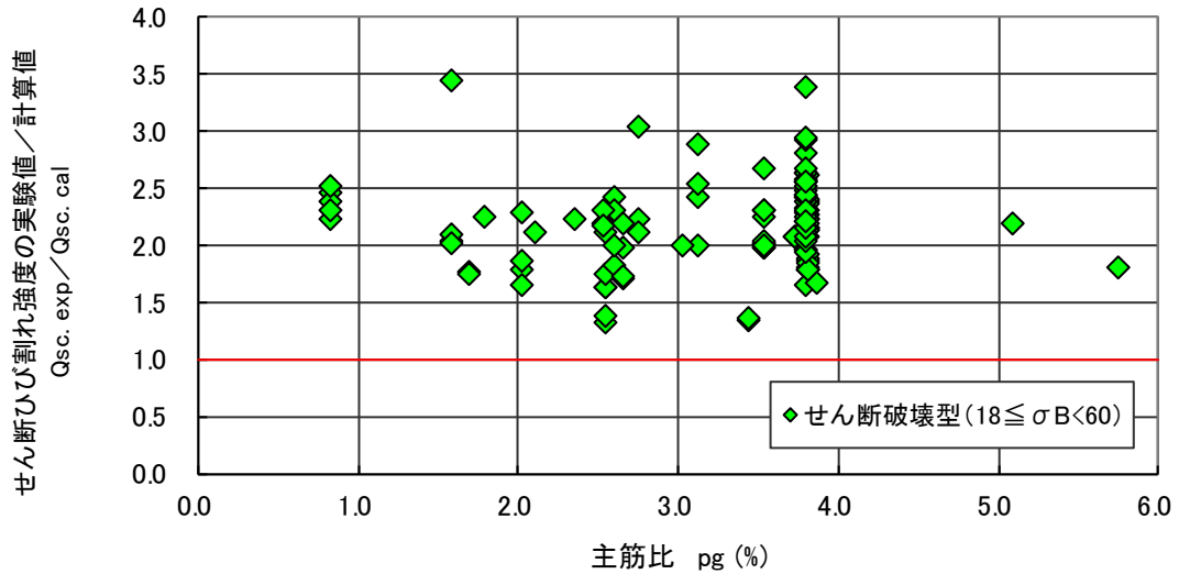
図 4.6.22 せん断ひび割れ強度 (実験値/計算値) - 主筋比関係 (せん断破壊型)
