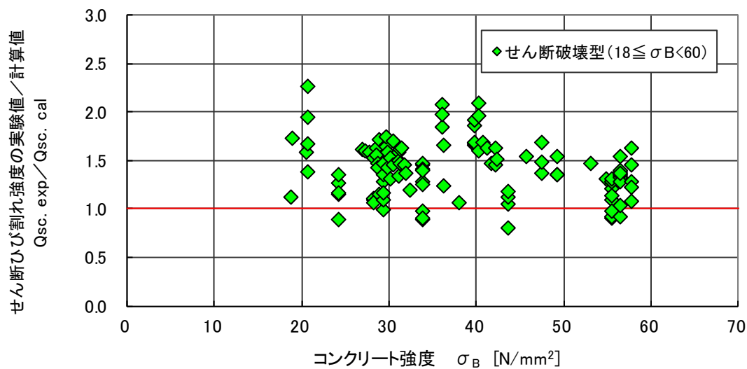
図 4.6.14 せん断ひび割れ強度（実験値／計算値）－コンクリート強度関係（せん断破壊型）
