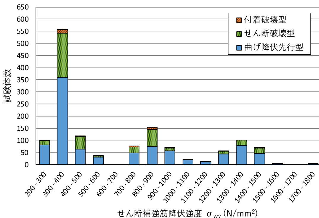
図 4.2.8 収集データの頻度分布 (せん断補強筋強度) (横軸は区間下限値以上から区間上限値未満)
