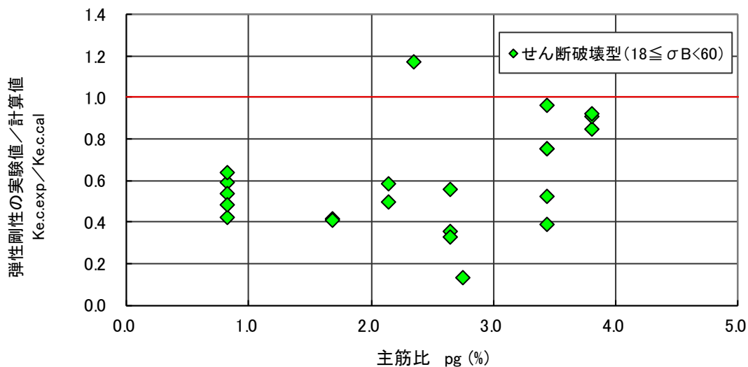
図 4.6.10 弾性剛性（実験値／計算値）－主筋比関係（せん断破壊型）
