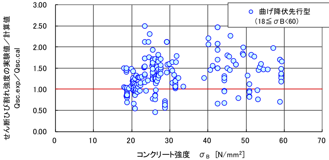
図 4.5.15 セン断ひび割れ強度（実験値／計算値）－コンクリート強度関係（曲げ降伏先行型）
