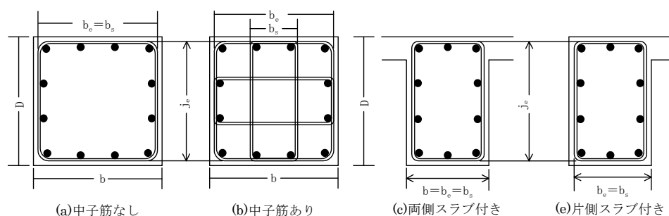
柱または梁の断面図
