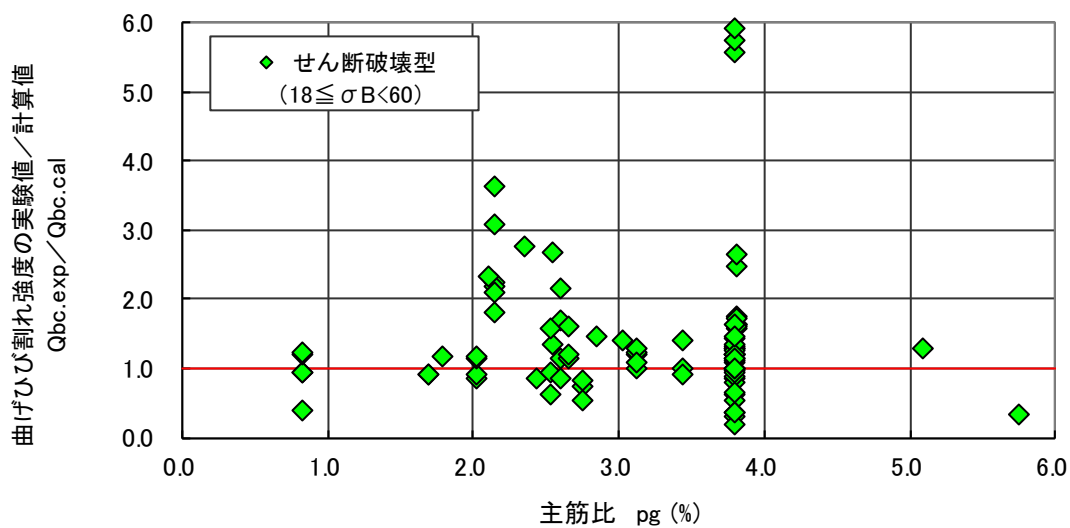
図 4.6.4 曲げひび割れ強度（実験値／計算値）－主筋比関係（せん断破壊型）
