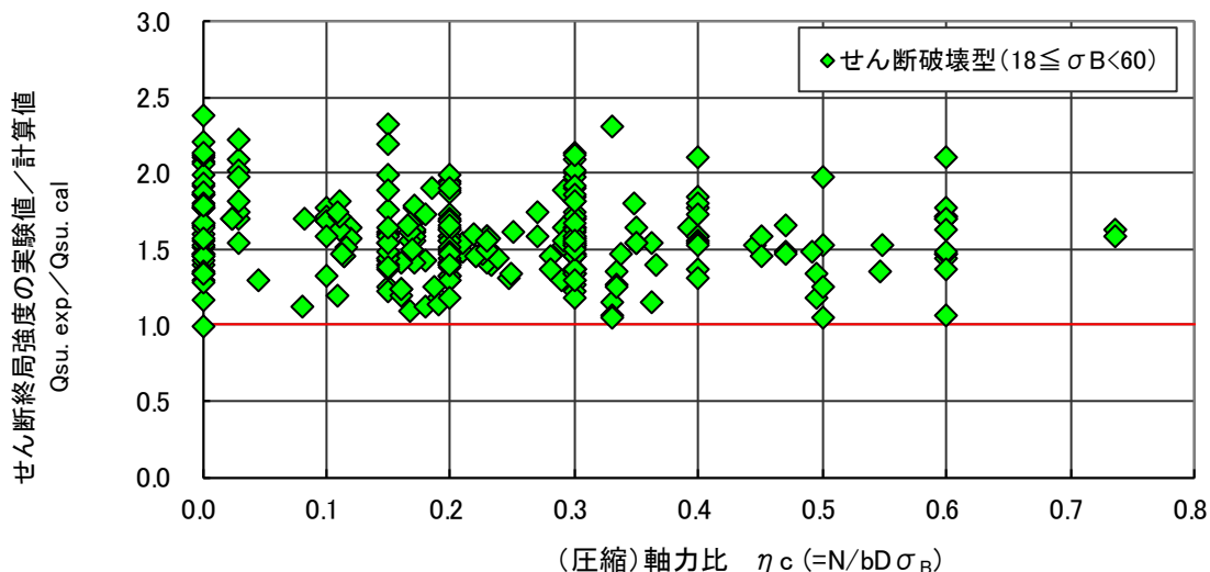
図 4.6.29 (実験値/計算値：基準下限式) - 圧縮軸力比関係 (せん断破壊型)
