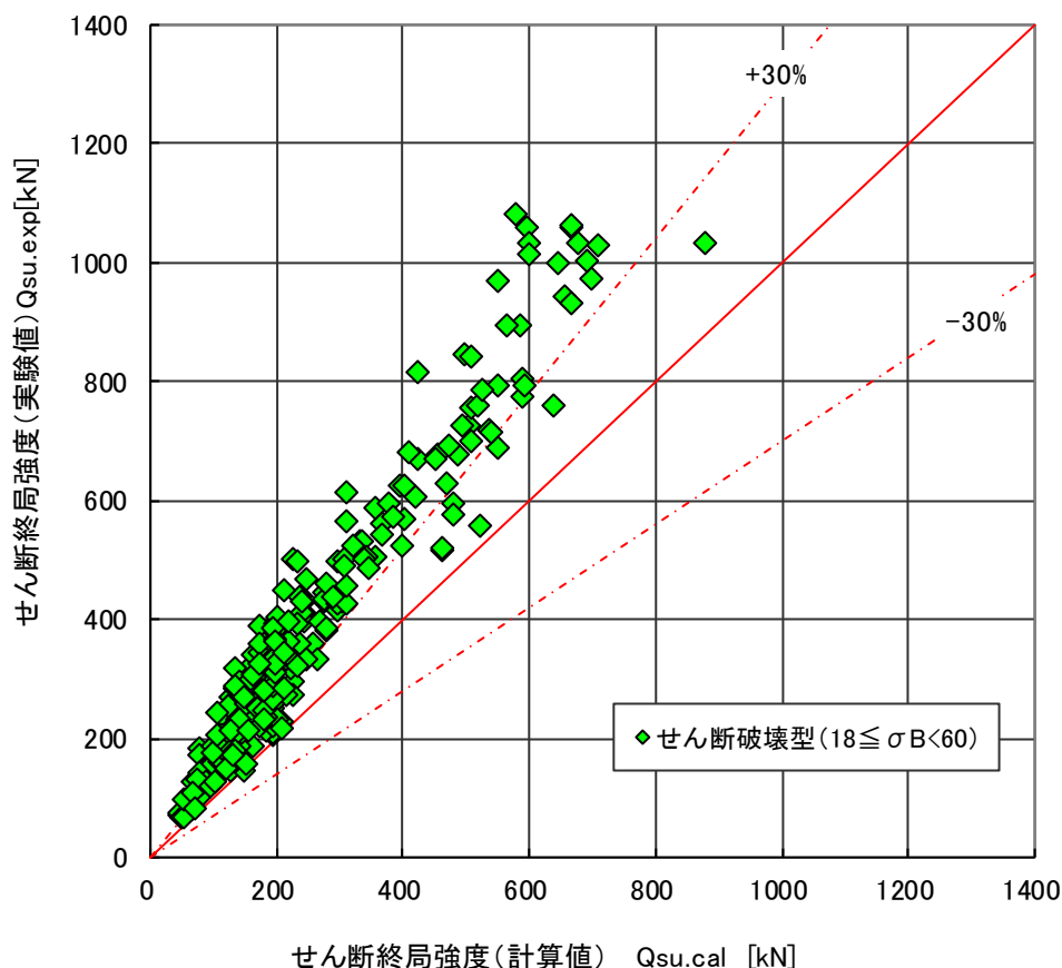
図 4.6.25 せん断強度の実験値と計算値（下限式）の比較（せん断破壊型）
