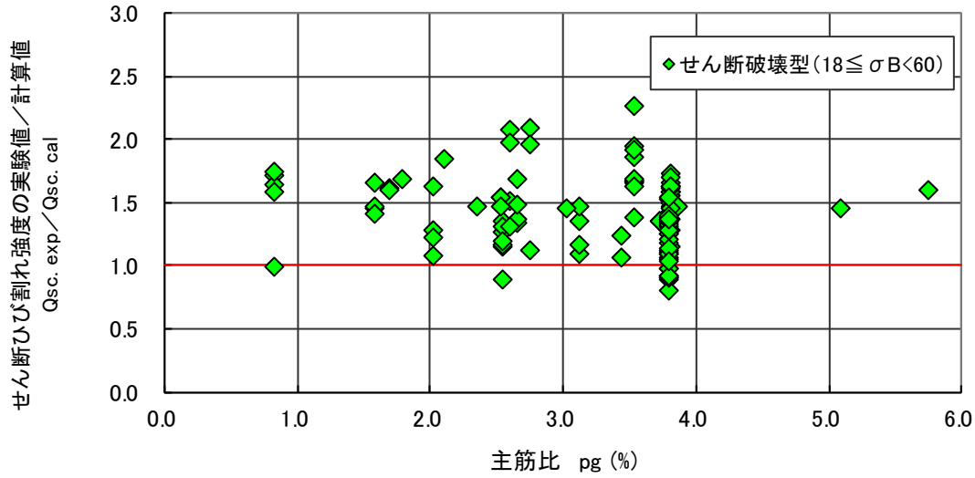
図 4.6.16 せん断ひび割れ強度（実験値／計算値）－主筋比関係（せん断破壊型）
