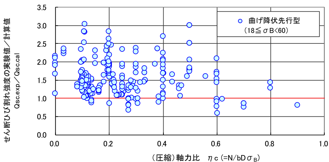
図 4.5.25 せん断ひび割れ強度（実験値／計算値）－圧縮軸力比関係（曲げ降伏先行型）
