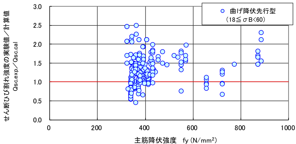
図 4.5.18 せん断ひび割れ強度（実験値／計算値）－主筋降伏強度関係（曲げ降伏先行型）
