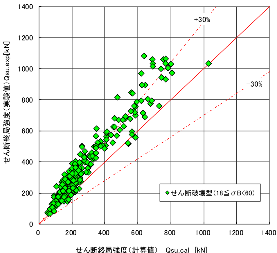
図 4.6.32 せん断強度の実験値と計算値（平均値式）の比較（せん断破壊型）
