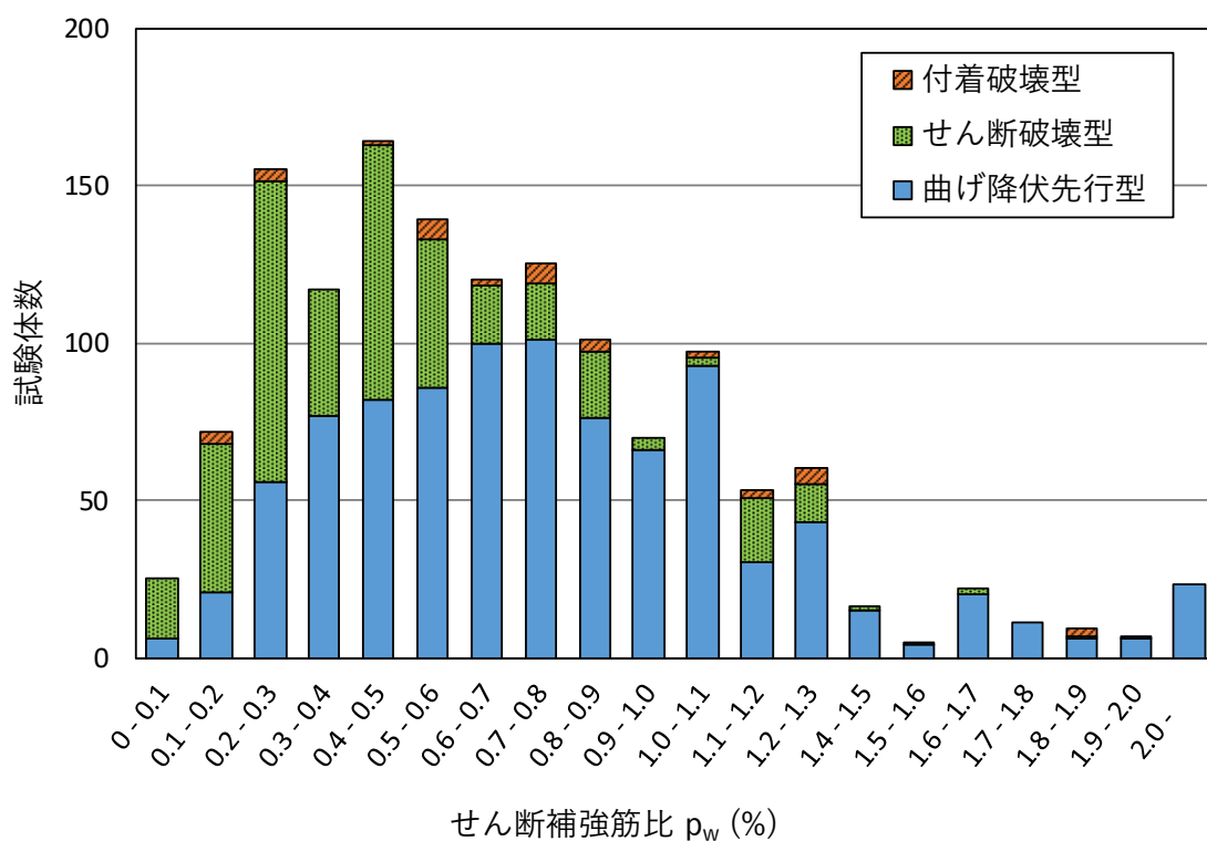
図 4.2.9 収集データの頻度分布 (せん断補強筋比) (横軸は区間下限値以上から区間上限値未満)
