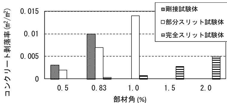
図 A-5 非耐力壁部材の部材角—コンクリート剥落率関係
