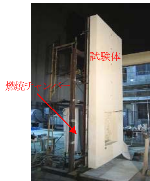
図 4 実験装置
