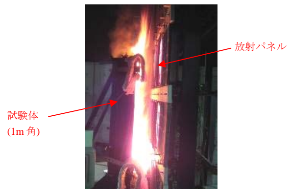
図 3 ICAL 試験の様子
