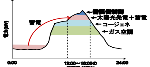
＜セントラル熱源システム＞
