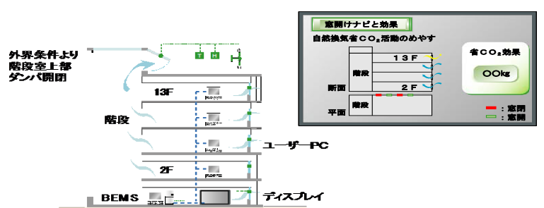
自然換気システム概念図
