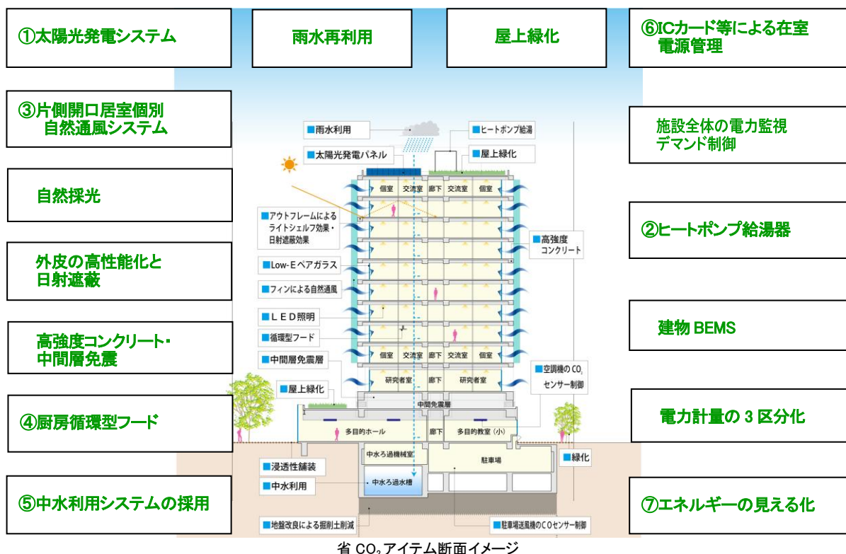
省 CO 2 アイテム断面イメージ
