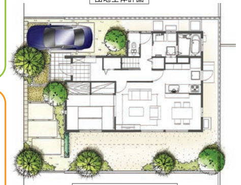
1階平面図(参考プラン)
